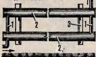
ГЛАДКОТРУБНЫЙ РЕГИСТР
