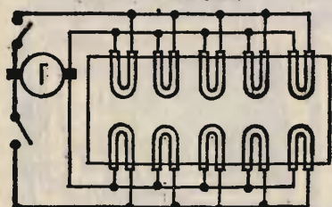
ЭЛЕКТРОСХЕМА
