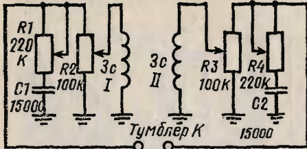
темброблок
